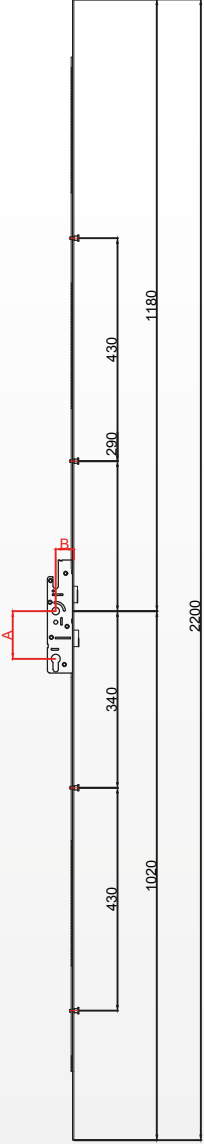
2200 Çift Tırtırlı Kilitli İspanyolet
