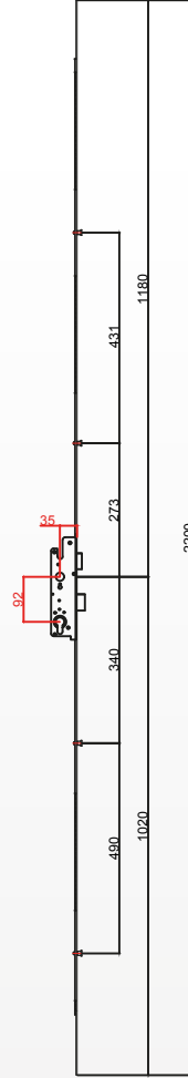
2200/92-35 Barelden Tahrirli Kilitli İspanyolet
