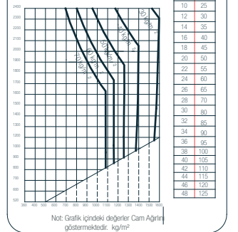
130 kg Yük Diyagramı
