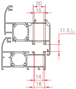
Uygulanabilir Kesit Detayları
