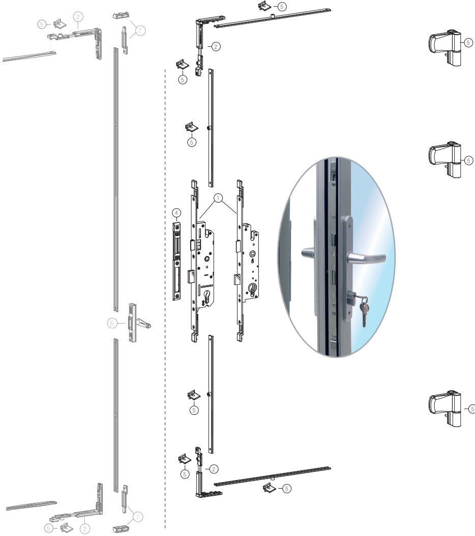
Koldan Kumandalı Çalıştırma Şekli
