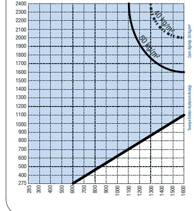
Cam Ağırlığı kg/m
