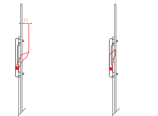
B - Kanca Kilitleme Pozisyonu A - Kanca Açık Pozisyonu
